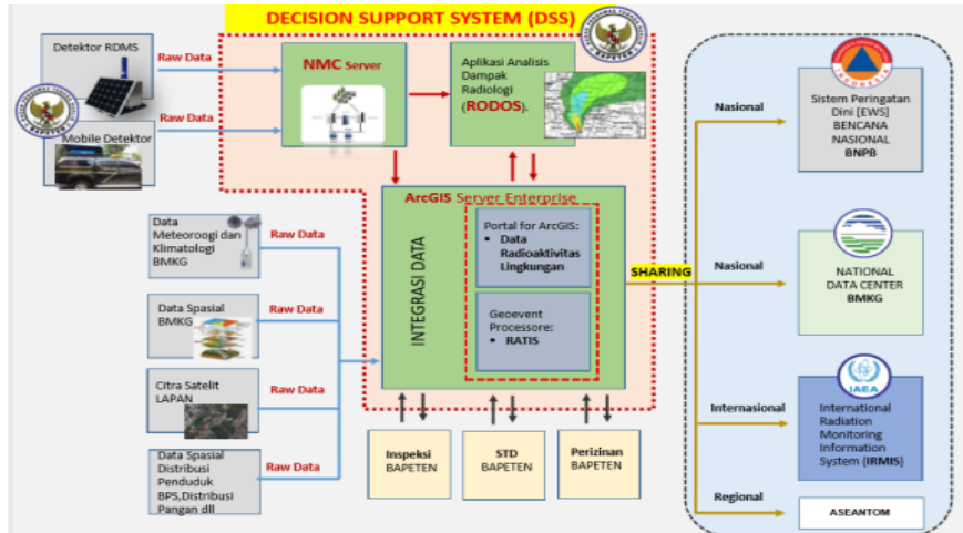
Gambar 7. Arsitektur I-RDMS
